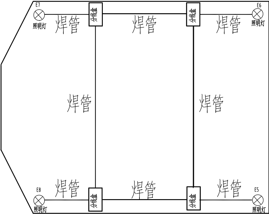
回转平台下方四角照明示意图
