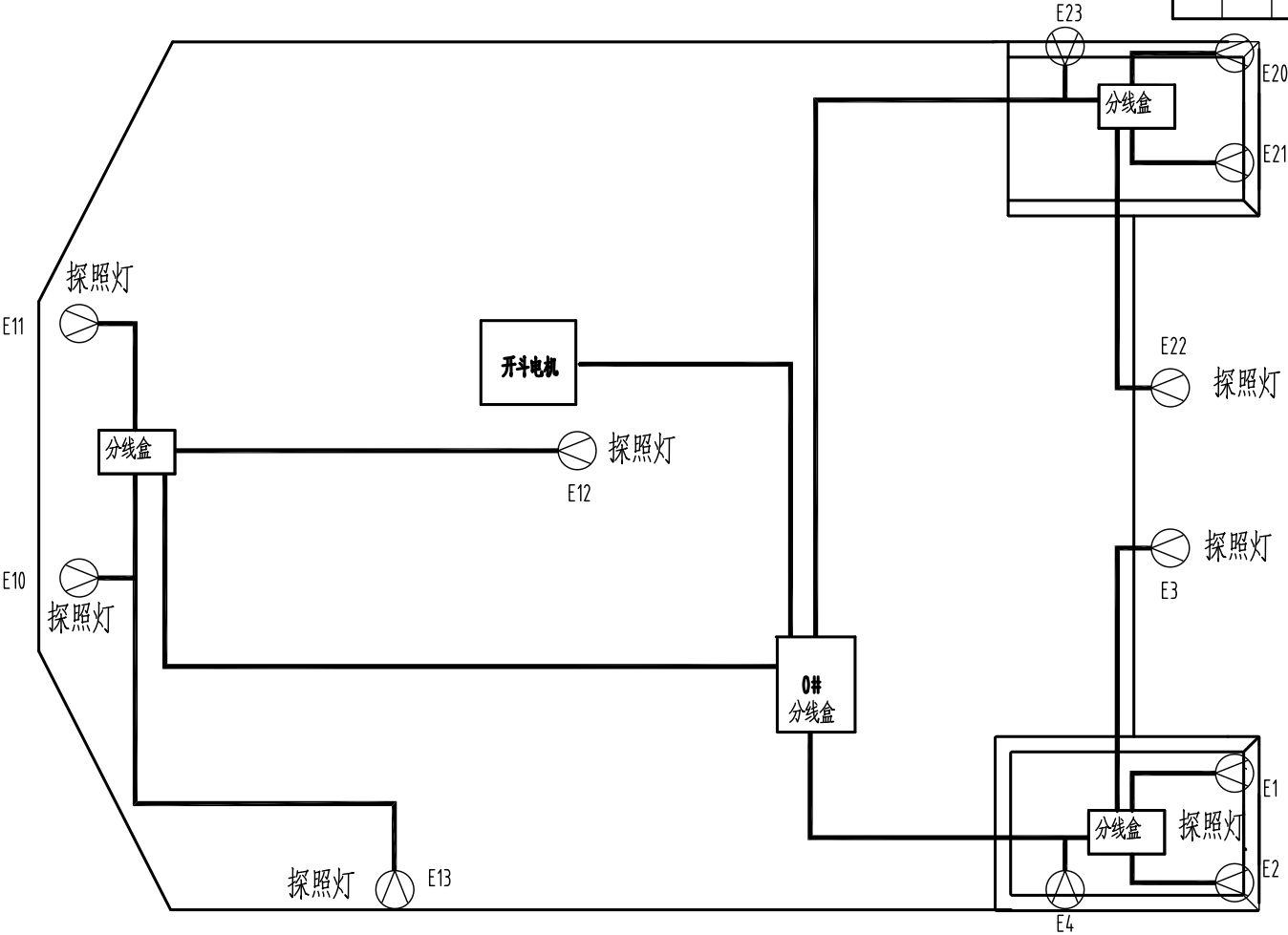
探照灯安转示意图
